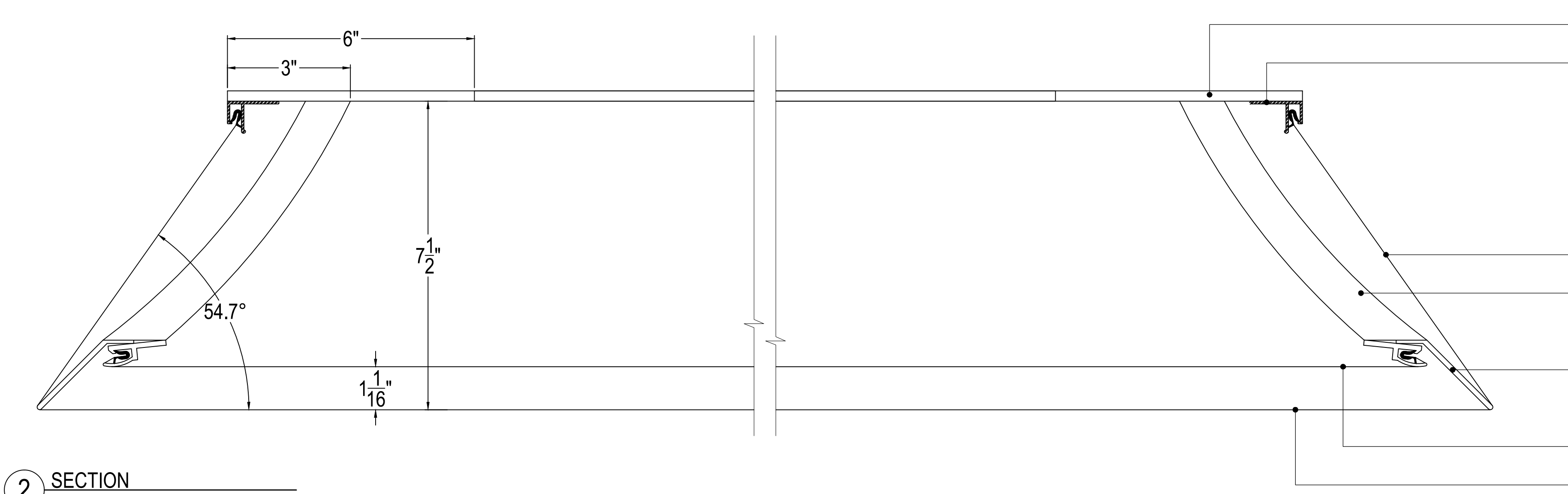
2 SECTION SCALE: 6" = 1'-0"
