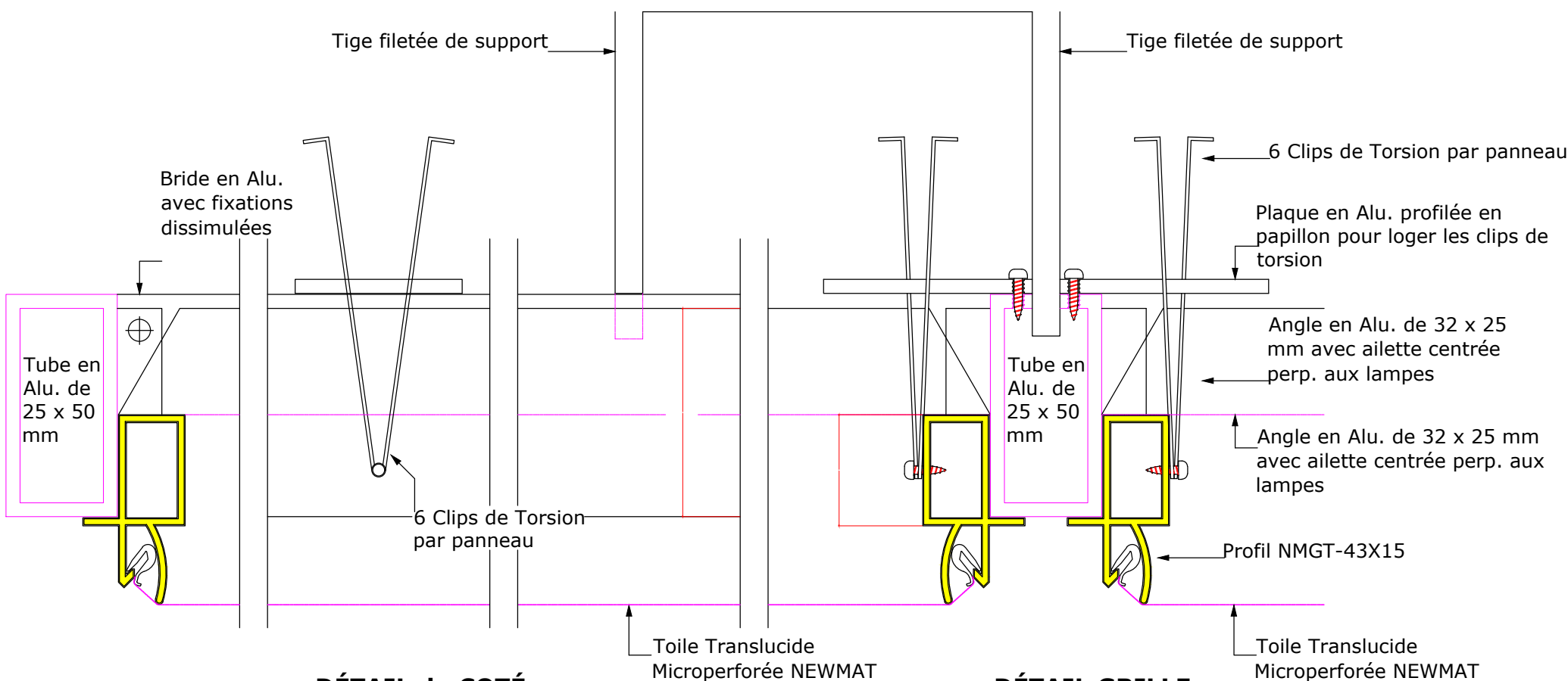
NEWMAT îlot avec panneaux acoustiques, translucides et accessibles - Détail CCA-TAP
