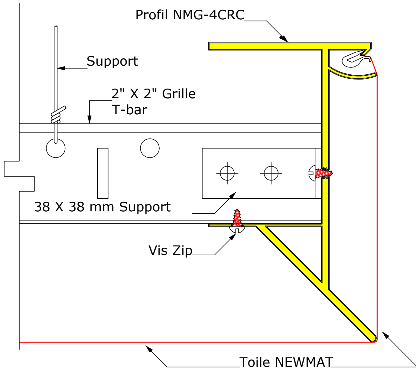
Panneau de plafond avec profil NMG-4CRC monté sur 2"X2" Grille T-Bar - Détail CRC-24
