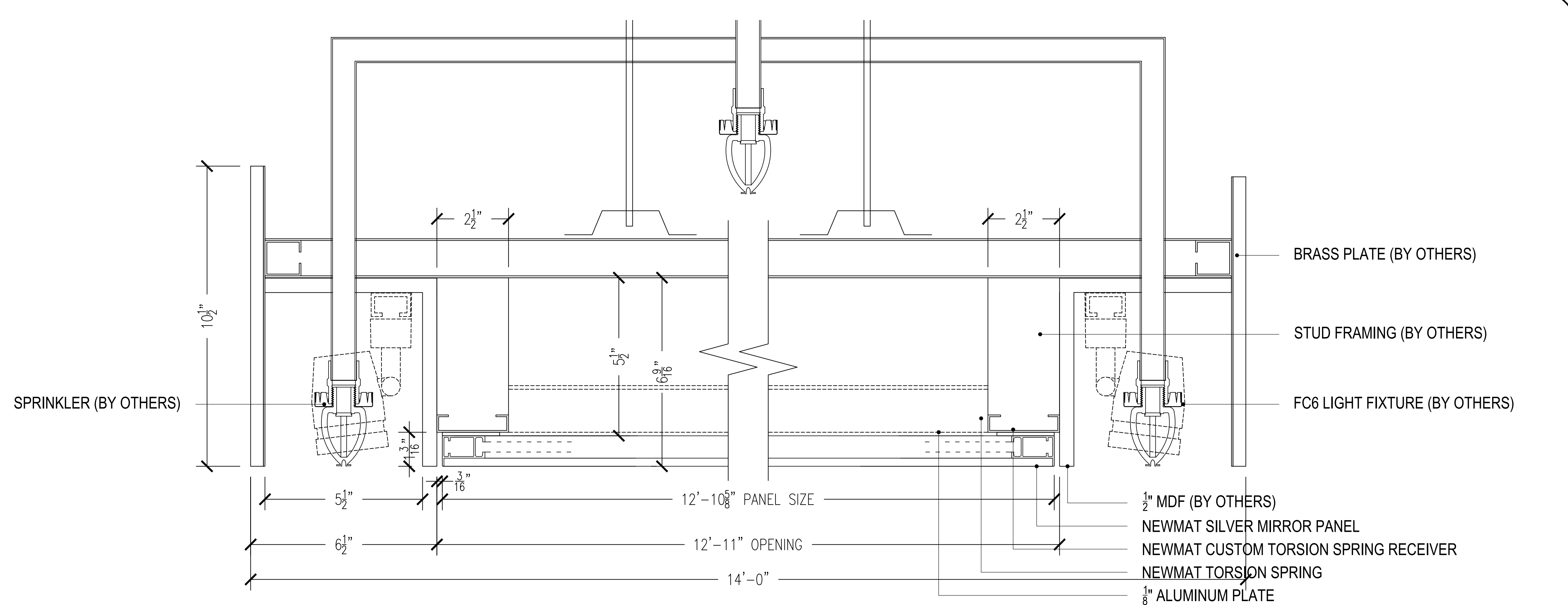
2 CEILING SECTION SCALE: 6" = 1'-0"
